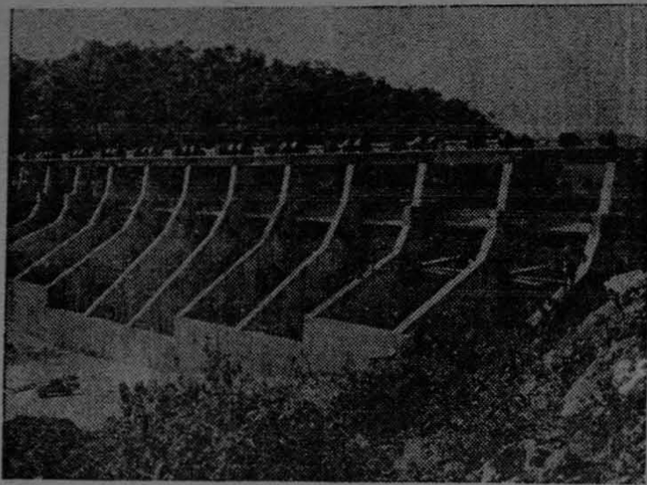
La gran presa Presidente Alemán, construida sobre el río Tonto, en la Cuenca del Papaloapan, y una de las mayores del país. La cortina tiene una altura máxima de 75 metros y 830 metros de extensión lineal.
